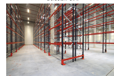
Budowa hali w Śląskim Centrum Logistycznym dla BIK Sosnowiec 2 Sp. z o.o.
