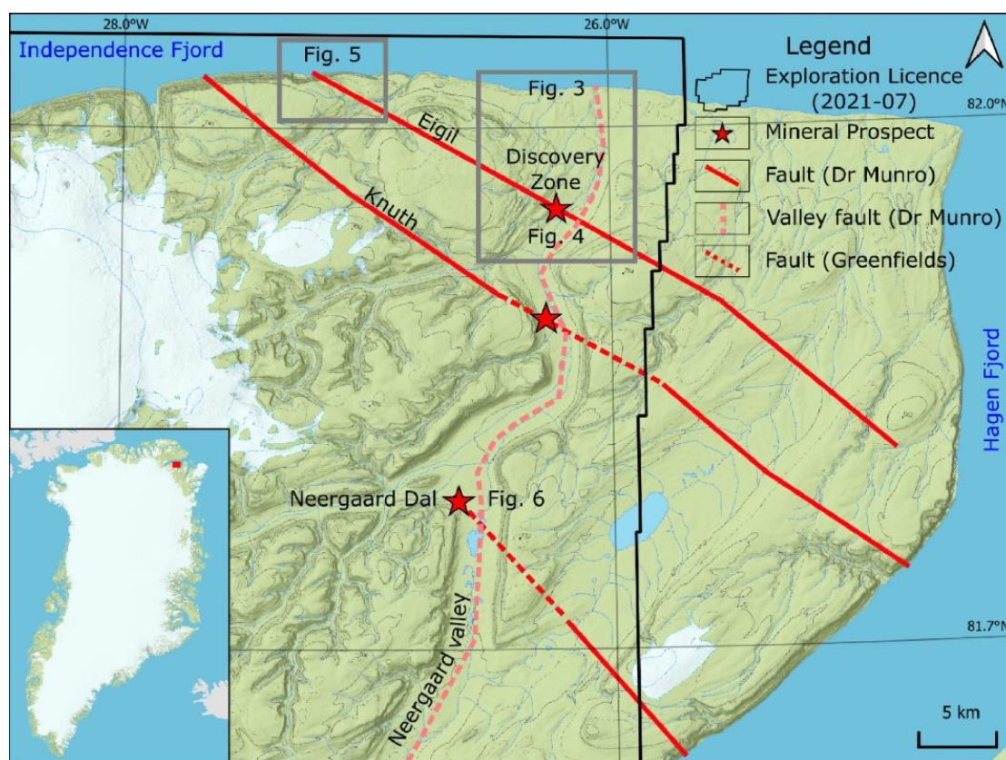
Rys. 1: Znaczące uskoki wsteczne zidentyfikowane w ARC (Uwaga: podczas gdy ruch wsteczny jest ograniczony, ruch boczny/przesuwczy jest niepewny)
