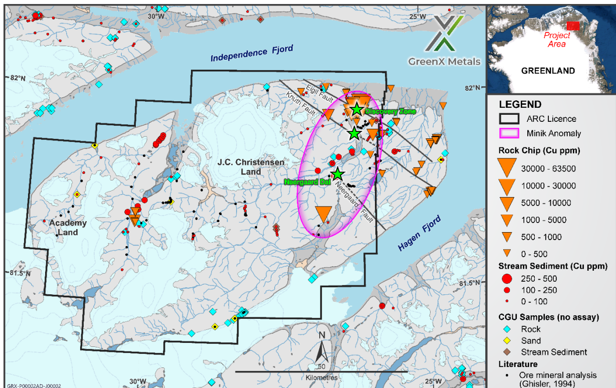
Rys. 2: Obszar objęty koncesją ARC przedstawiający geochemię historyczną, Anomalię Minik i zidentyfikowane uskoki
